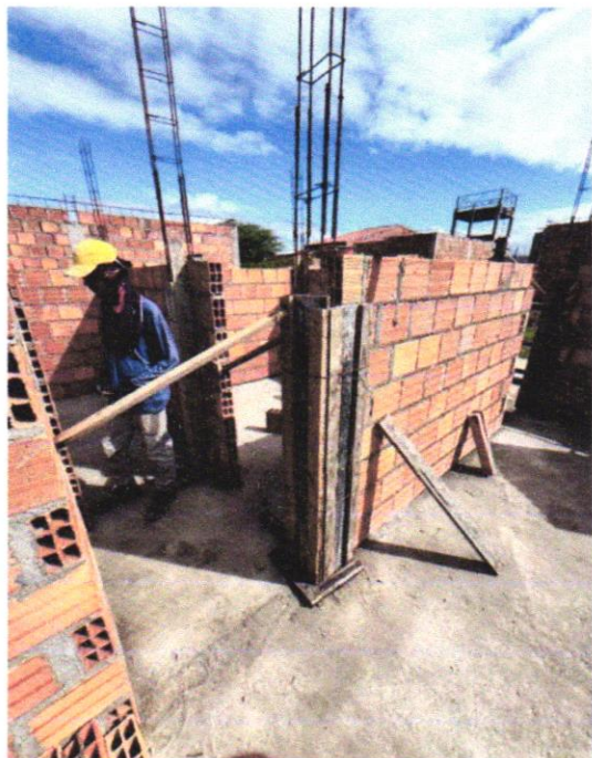
ARMAÇÃO DE PILAR
